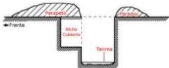
TRINCHERA DE APOYO / RESERVA
